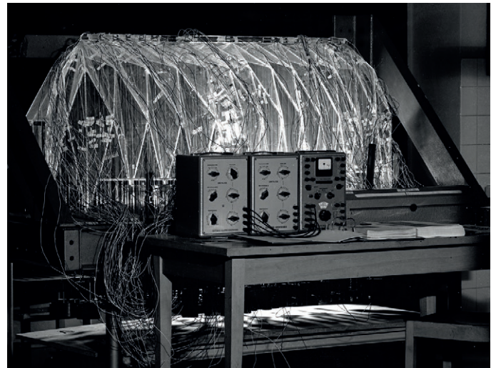
Stefan Polónyi: Statisches Versuchsmodell aus Acrylglas von St. Paulus, Neuss zur Dehnungsmessung am Institut für Modellstatik der Technischen Universität Berlin. o.D.
